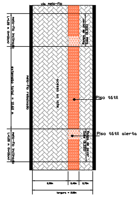
Acesso ao Lote Industrial - Passeio 2,20 metros - Planta Sem escola
