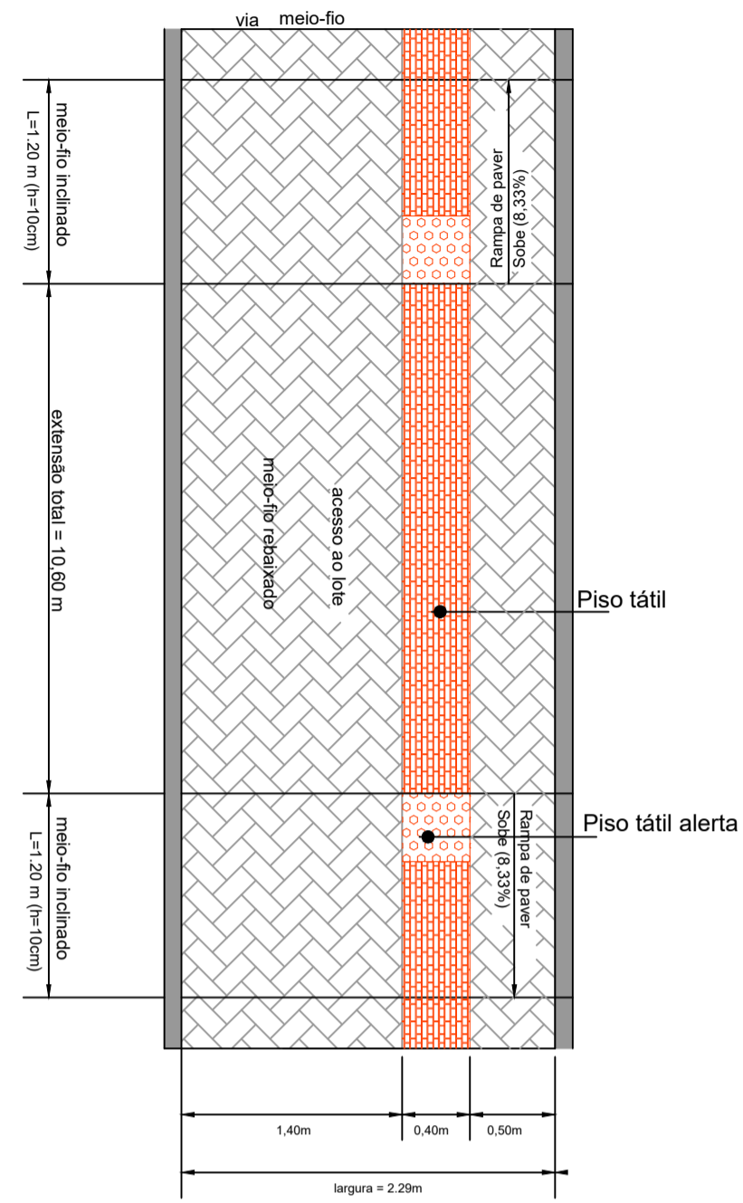
Acesso ao Lote Industrial - Passeio 2,30 metros - Planta Sem escala
