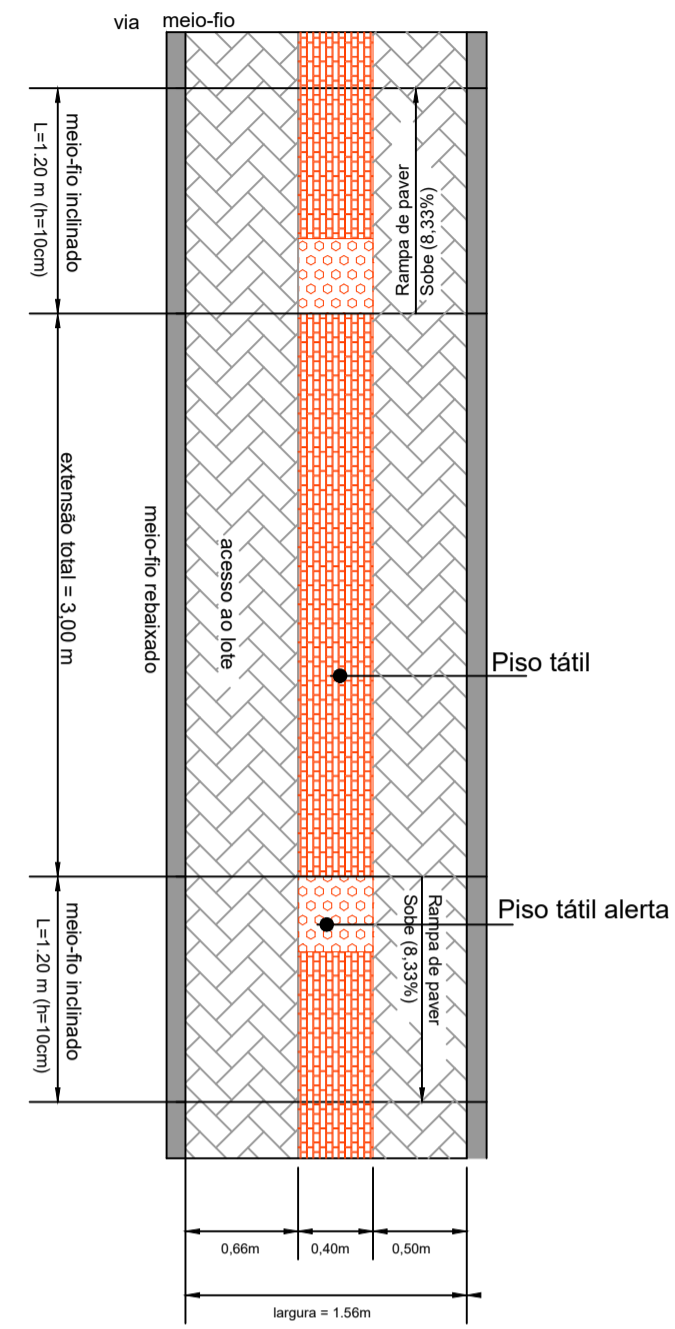
Acesso ao Lote Passeio 1,56 metros - Planta Sem escala
