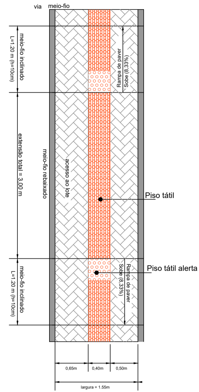
Acesso ao Lote Passeio 1,55 metros - Planta Sem escala
