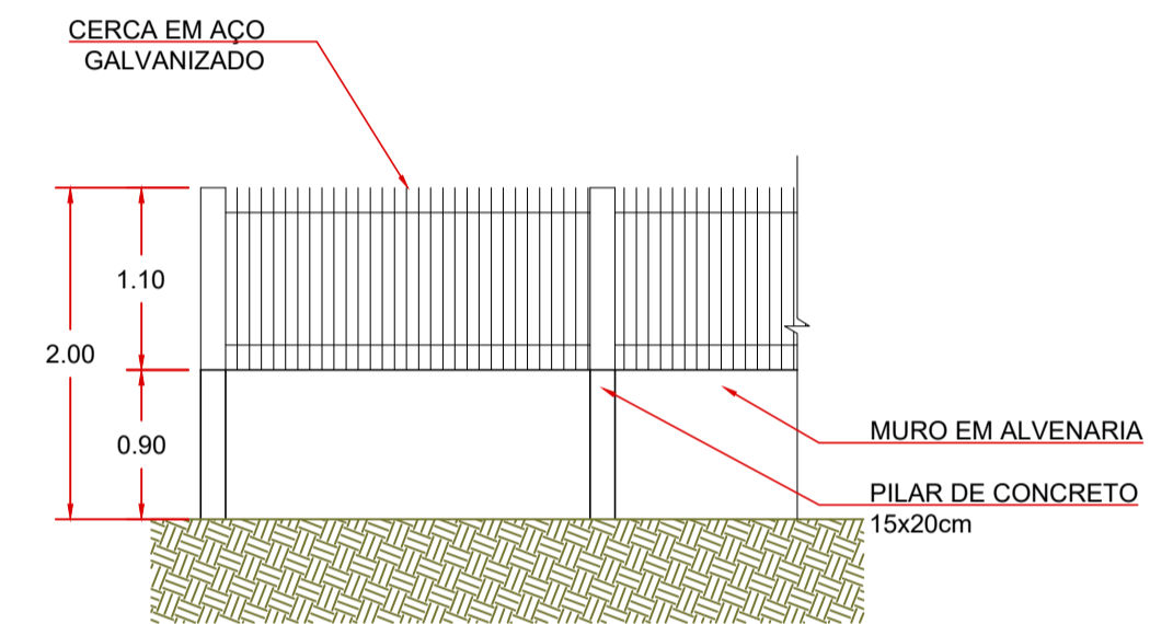
DETALHE 01 - MURETAS E CERCAMENTO ESC.: 1/50
