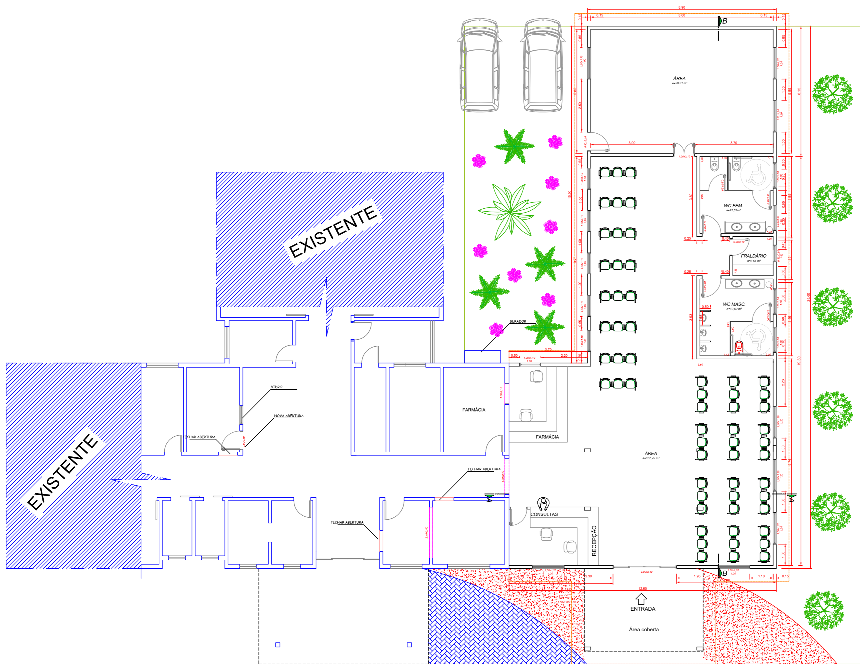
PLANTA DE SITUAÇÃO E LOCALIZAÇÃO ESC: 1/50
