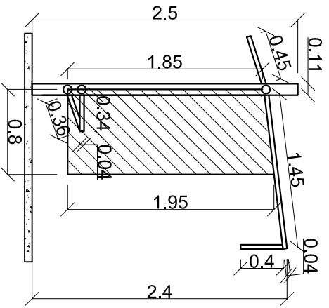
Croqui Abrigo de Ônibus Escala 1:50
